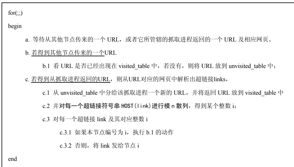
图 6-3 协调进程工作算法
