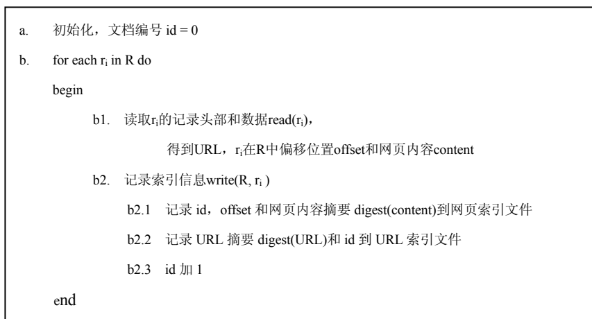
图 4-3 索引网页库算法
