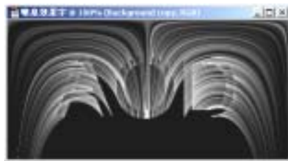
图 84.4 坐标变换
