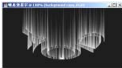
图 84.3 风效果
